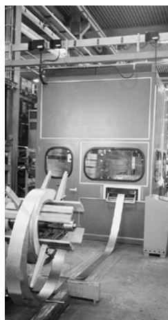
4 Incapsulamento integrale di una pressa automatica
